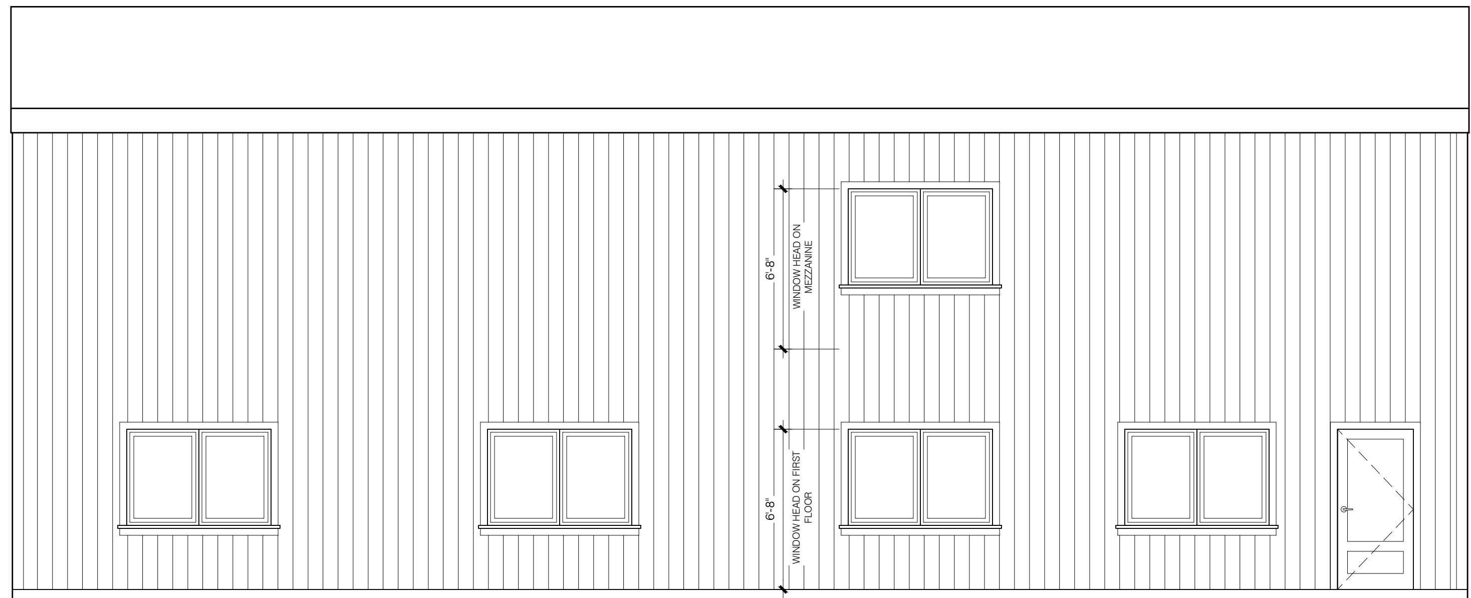
2 A3 SIDE ELEVATION SCALE: 1/4" = 1'-0"
